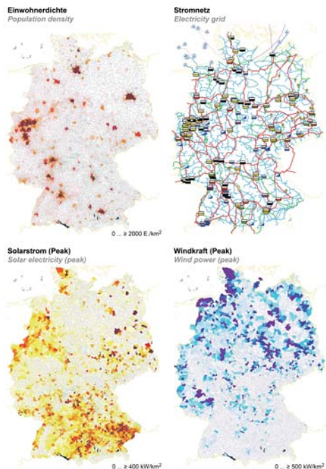
Stromnetz Deutschland – Erzeuger (EE, KW), Lasten und Netz The power grid in Germany – generation (renewable energy, power plants), loads and grid
